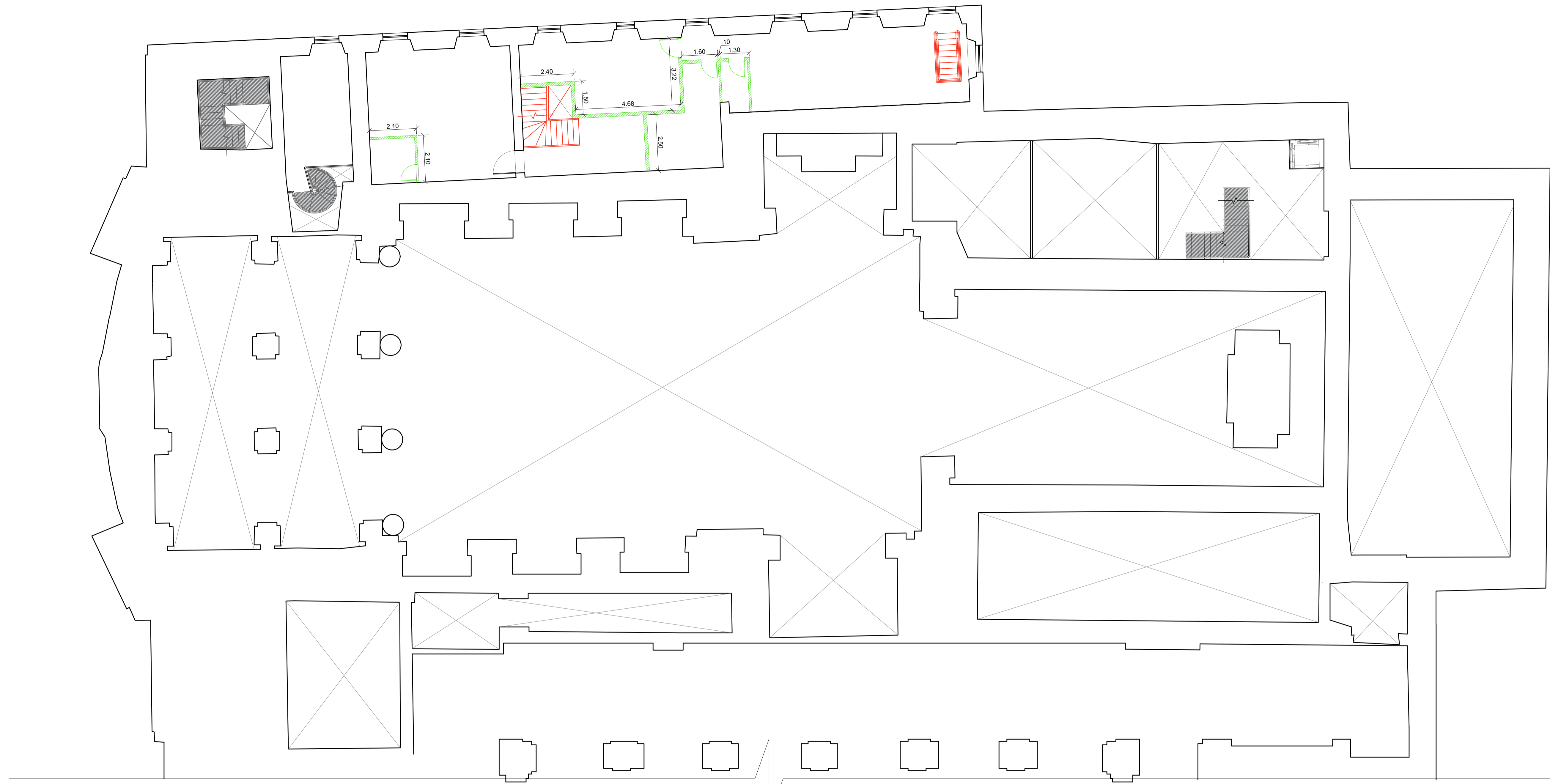
PLANTA DE DEMOLIÇÃO E CONSTRUÇÃO - PAV. INTERMEDIÁRIO ESC 1/100
