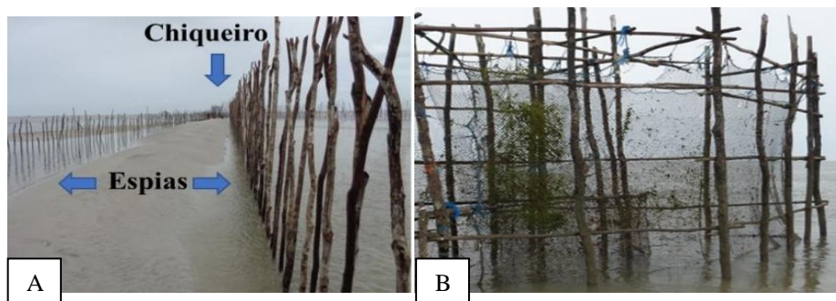
Figura 2: Compartimentos do curral
